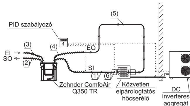
2. ábra. A HVM kísérleti mérőállás kapcsolási rajza
