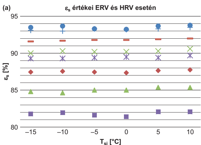
13. ábra Az ERV és HRV szenzibilis hatásfok (%) értékei a külső léghőmérséklet (°C) függvényében, különböző levegő térfogatáramok mellett, (a) téli időszak és (b) nyári időszak esetén
