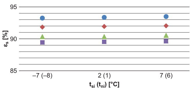
12. ábra A szenzibilis hatásfok (%) értékei a külső léghőmérséklet (°C) függvényében, különböző levegő térfogatáramok mellett
